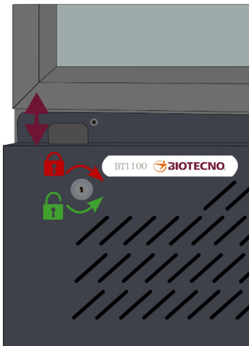
Figura 22-Sistema de fechamento da porta com chave.
