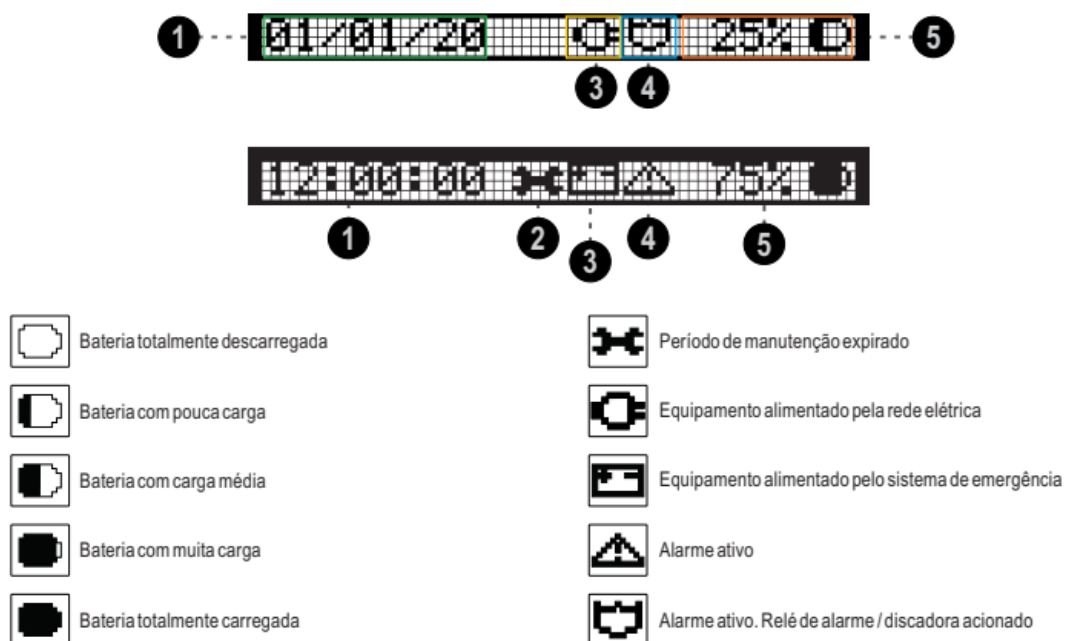
Figura 8-Barra de Status.
