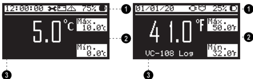
Figura 7-Tela Inicial
