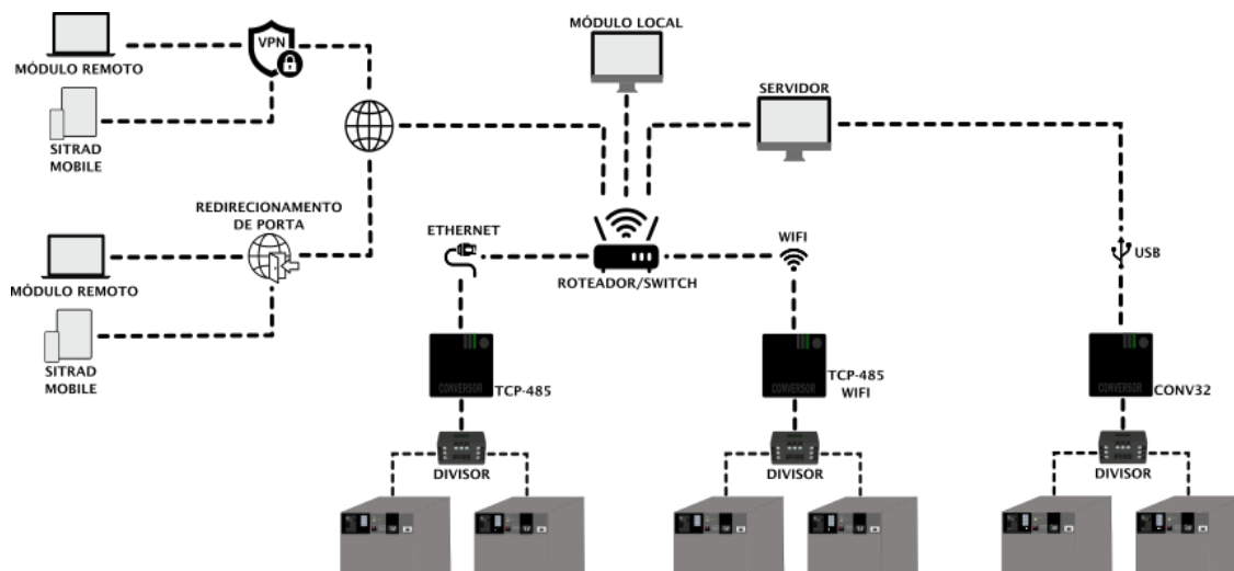
Figura 13-Topologia de Rede.
