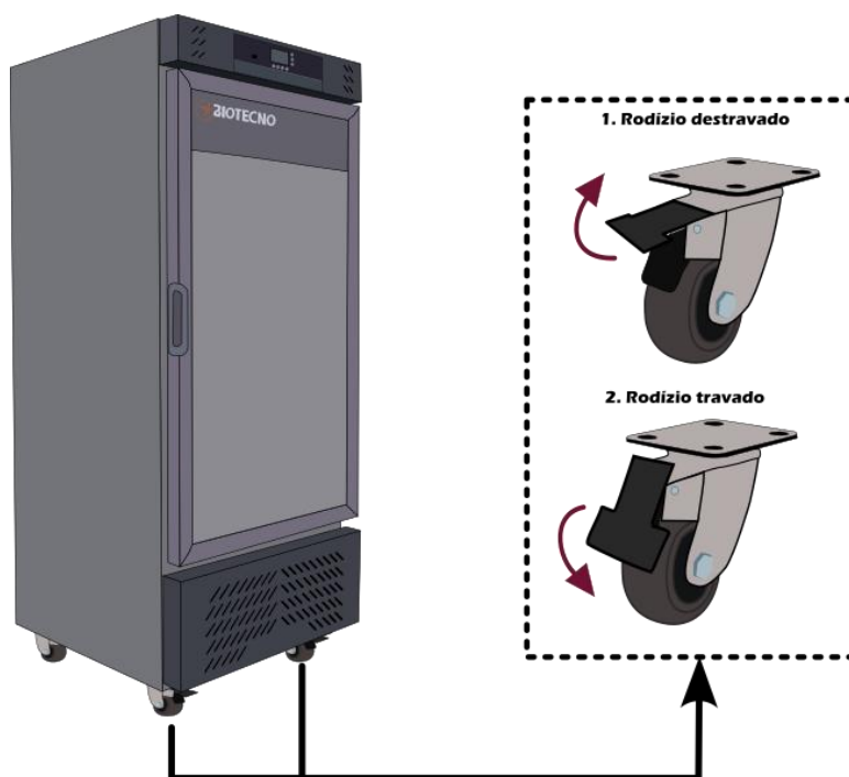
Figura 21-Instruções de travamento dos rodízios.
