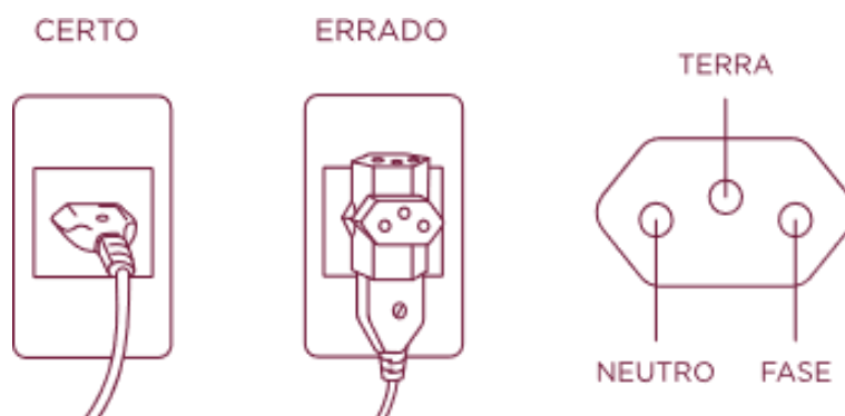
Figura 1-Especificações da tomada.
