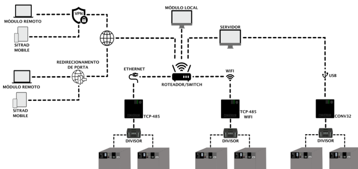
Figura 6-Topologia de Rede.
